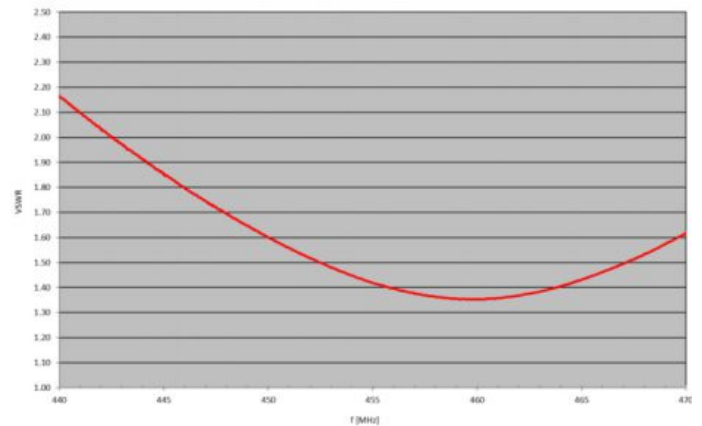
VSWR @ +45° input
